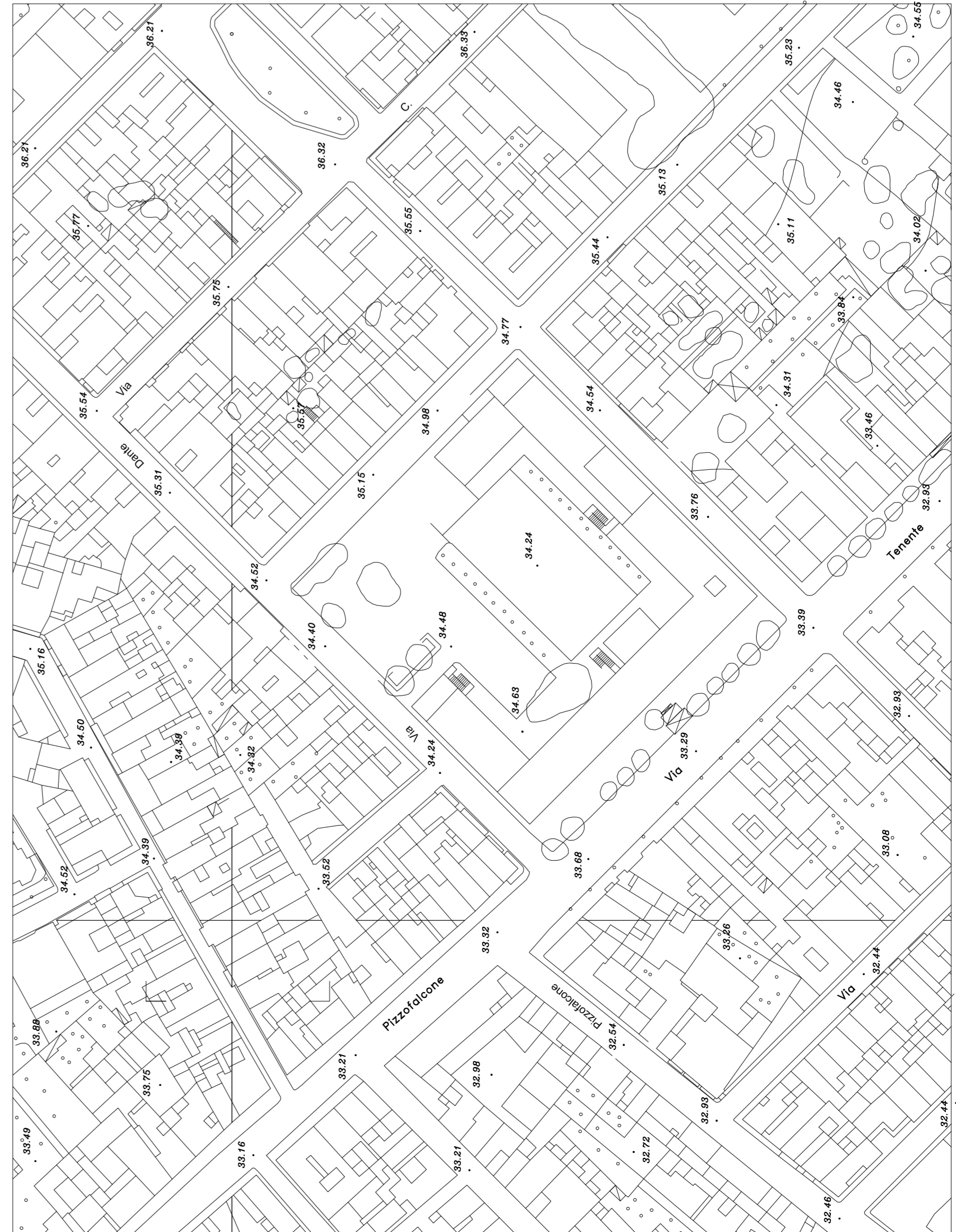
STRALCIO AEROFOTOGRAMMETRICO 1/1000
