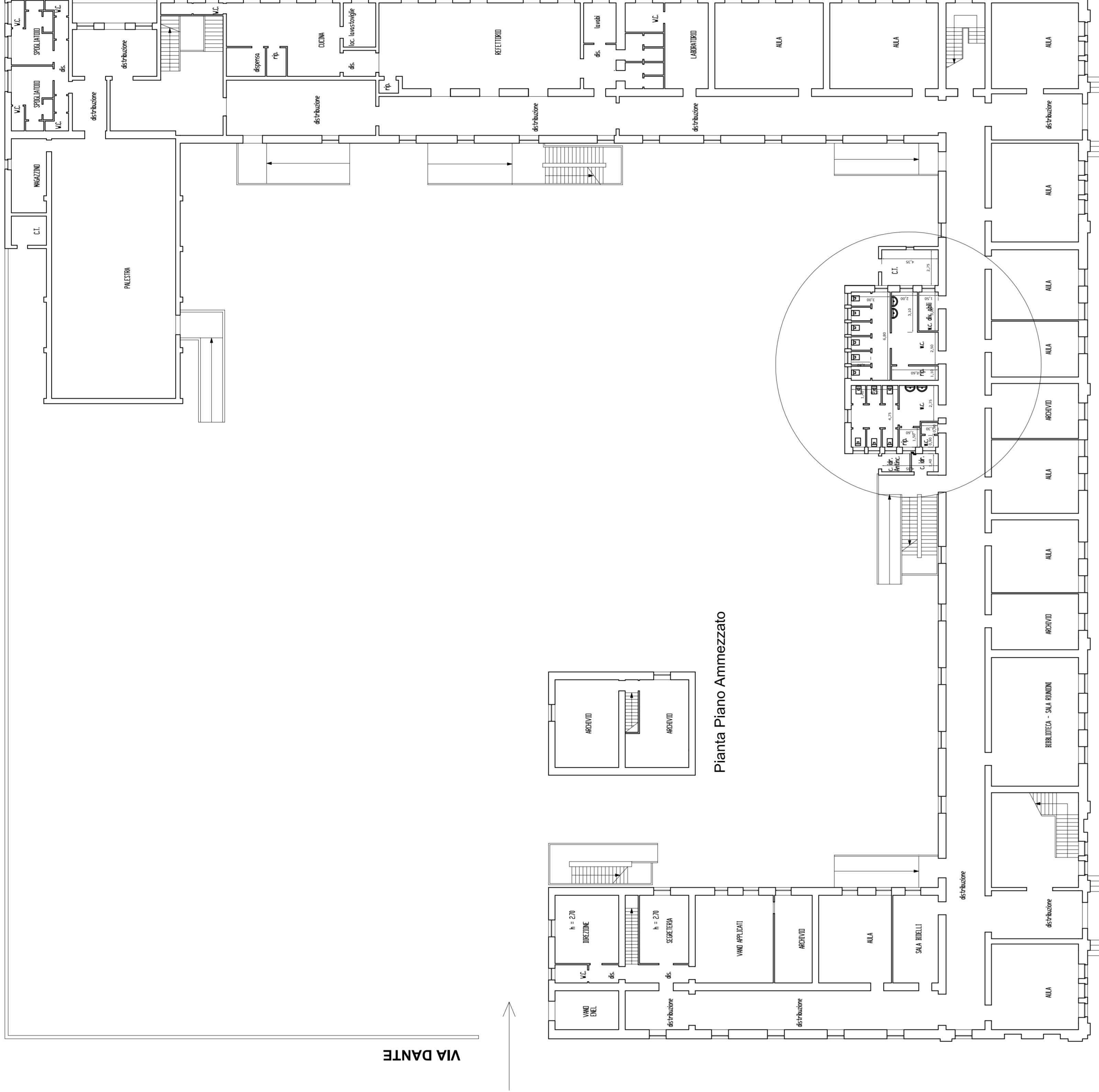
VIA TENENTE COLACI ADEGUAMENTO SERVIZI IGIENICI EDIFICIO SCOLASTICO DI VIA T. COLACI Polo 1° Pianta Piano Terra rapp. 1:200
