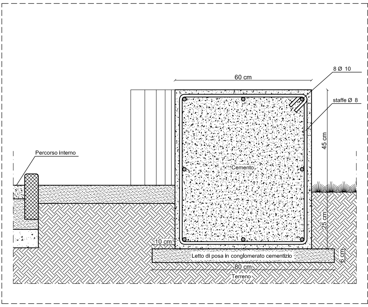
PARTICOLARE COSTRUTTIVO PANCHINA IN CEMENTO ARMATO - Scala 1:10
