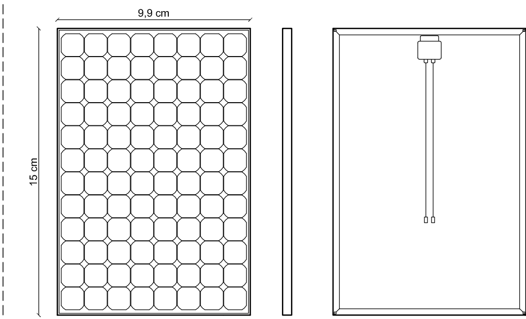
PALO DI ILLUMINAZIONE LED - Dettaglio Pannello Solare
