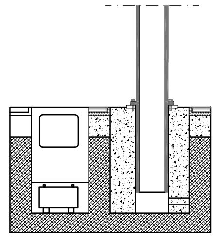
PALO DI ILLUMINAZIONE LED - Sezione Blocco di Fondazione
