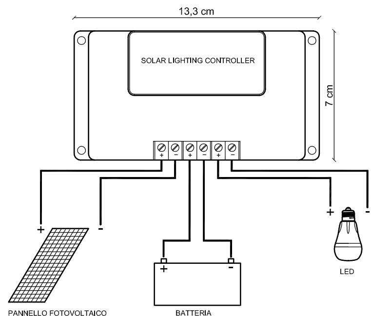
PALO DI ILLUMINAZIONE LED - Dettaglio Collegamento Controller
