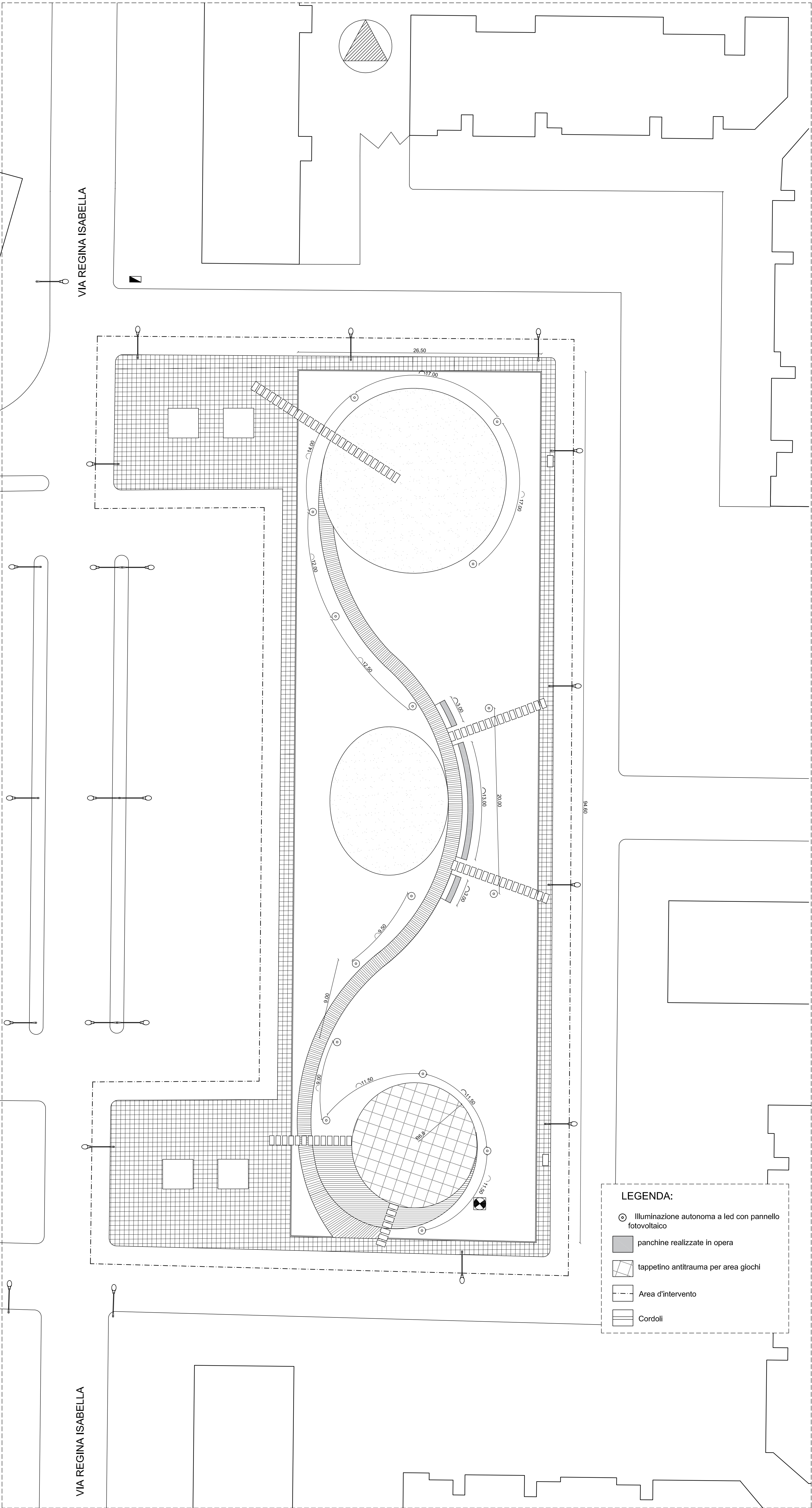
PLANIMETRIA DI PROGETTO, scala 1:200
