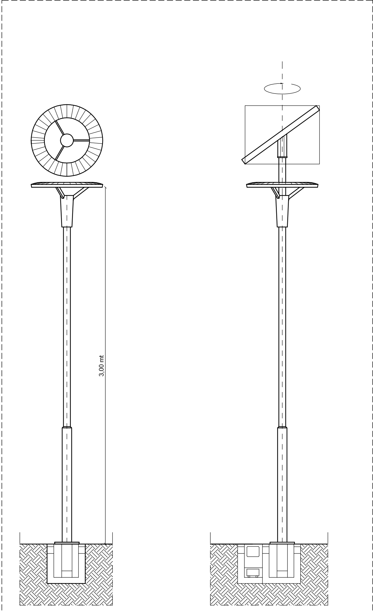
PALO DI ILLUMINAZIONE LED Sezione Frontale
