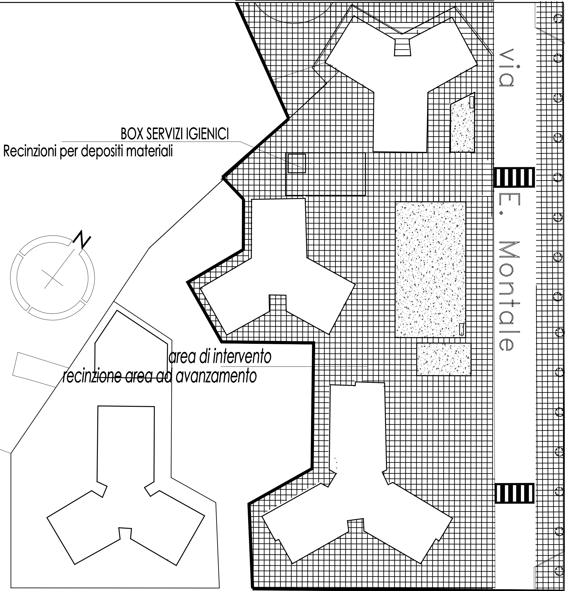
LAY-OUT DI CANTIERE
