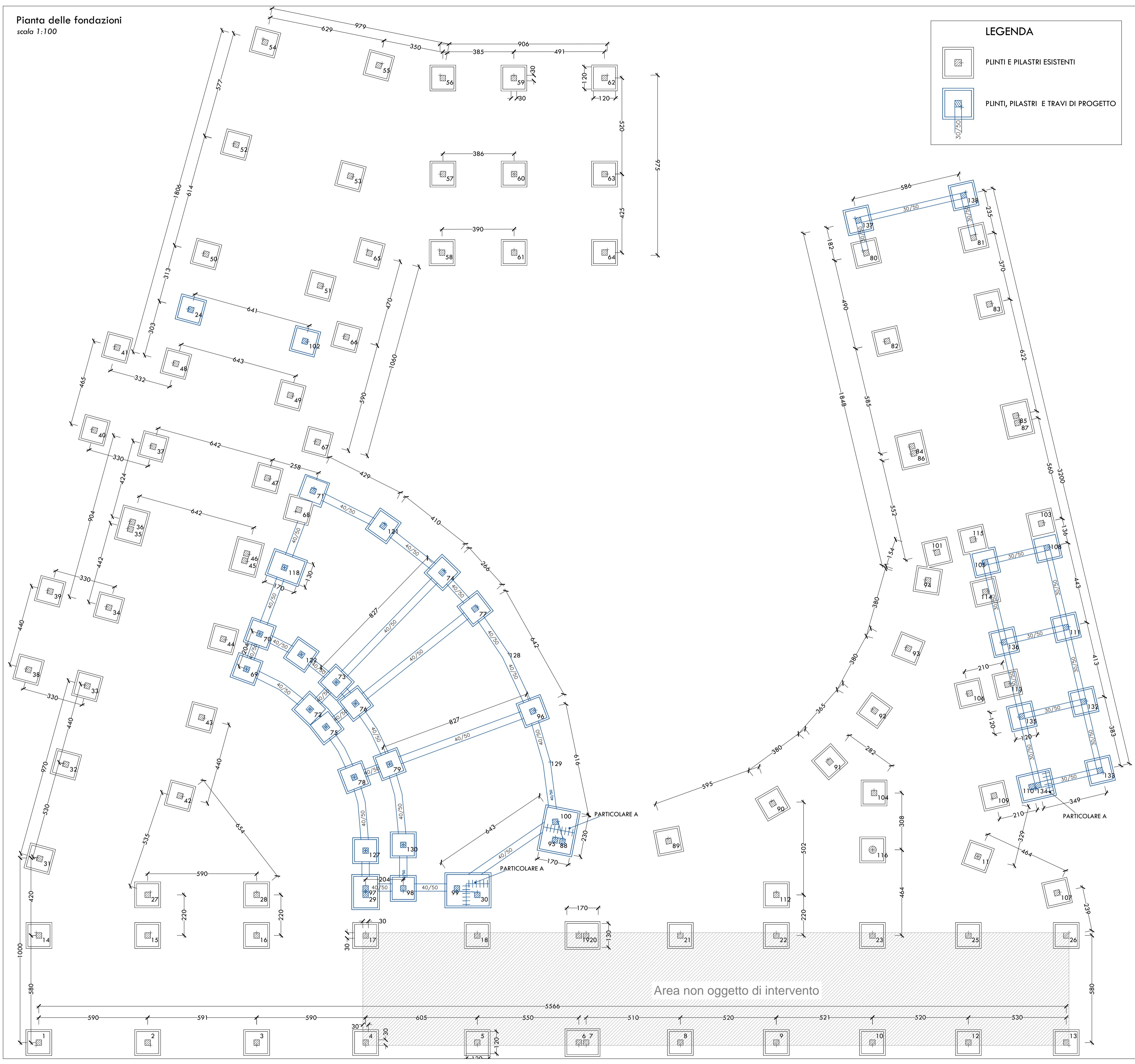
ZATTERA PLINTO scala 1:50
