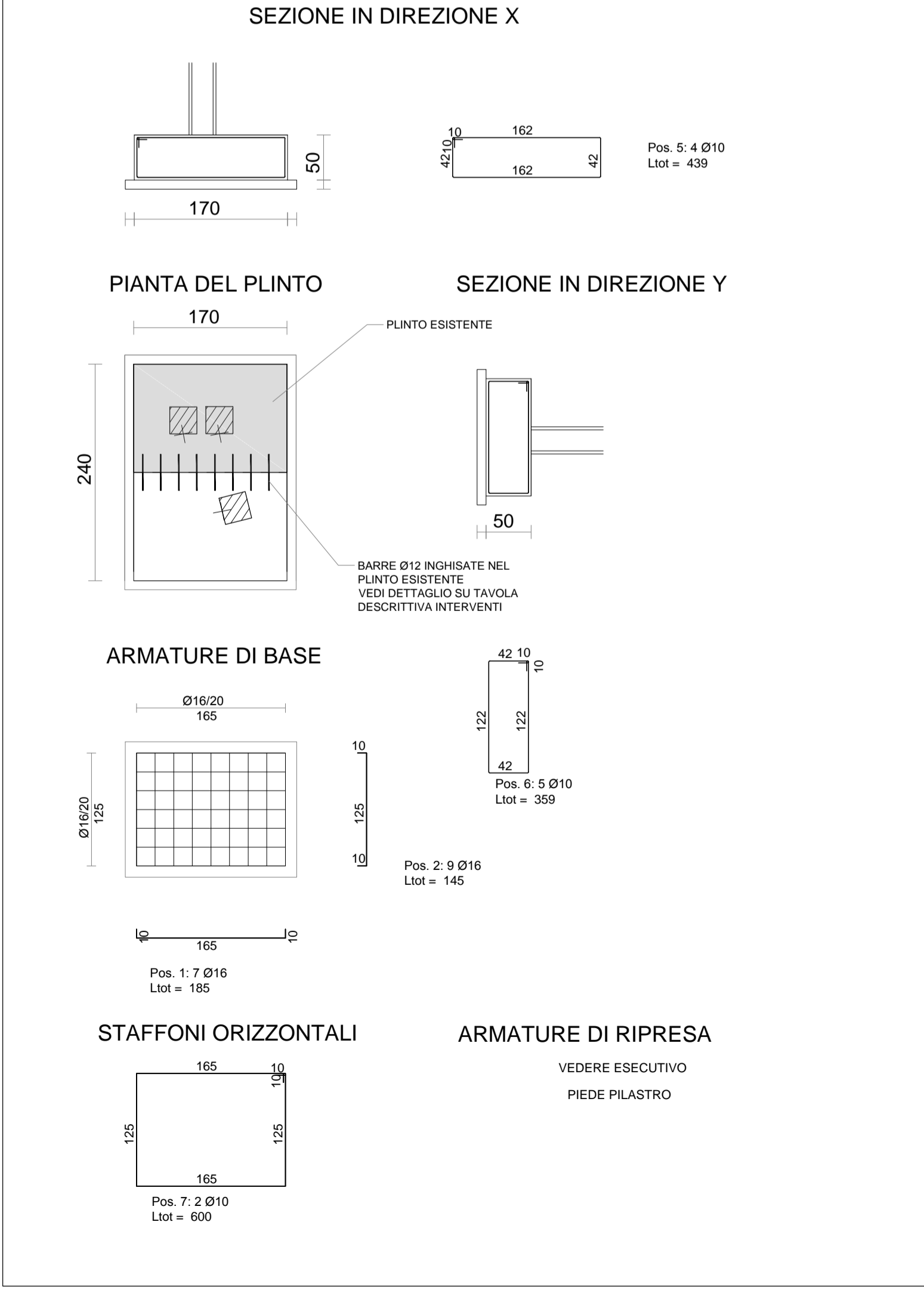
ZATTERA PLINTO N.ro 88-95-100 scala 1:50
