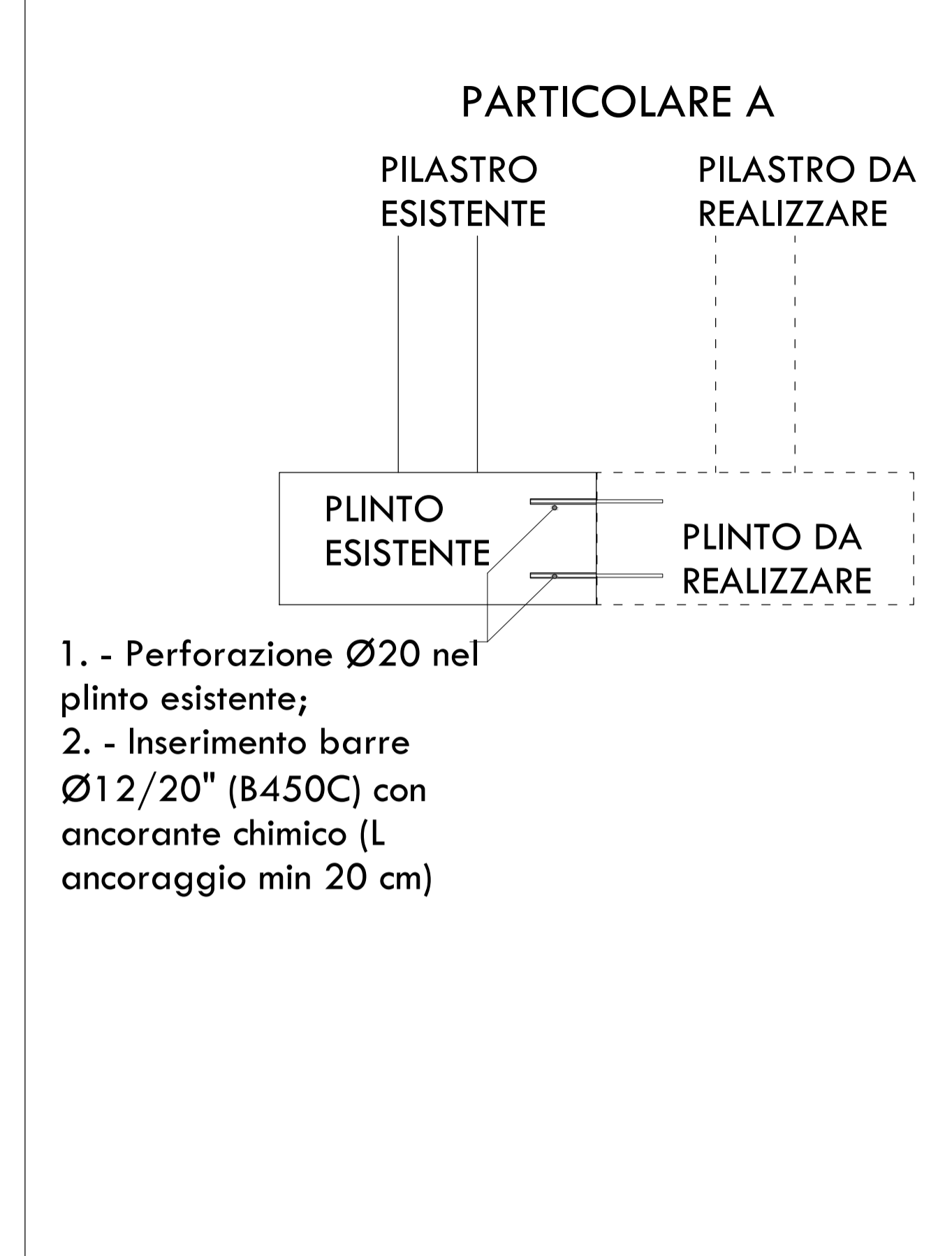
PARTICOLARE A scala 1:50
