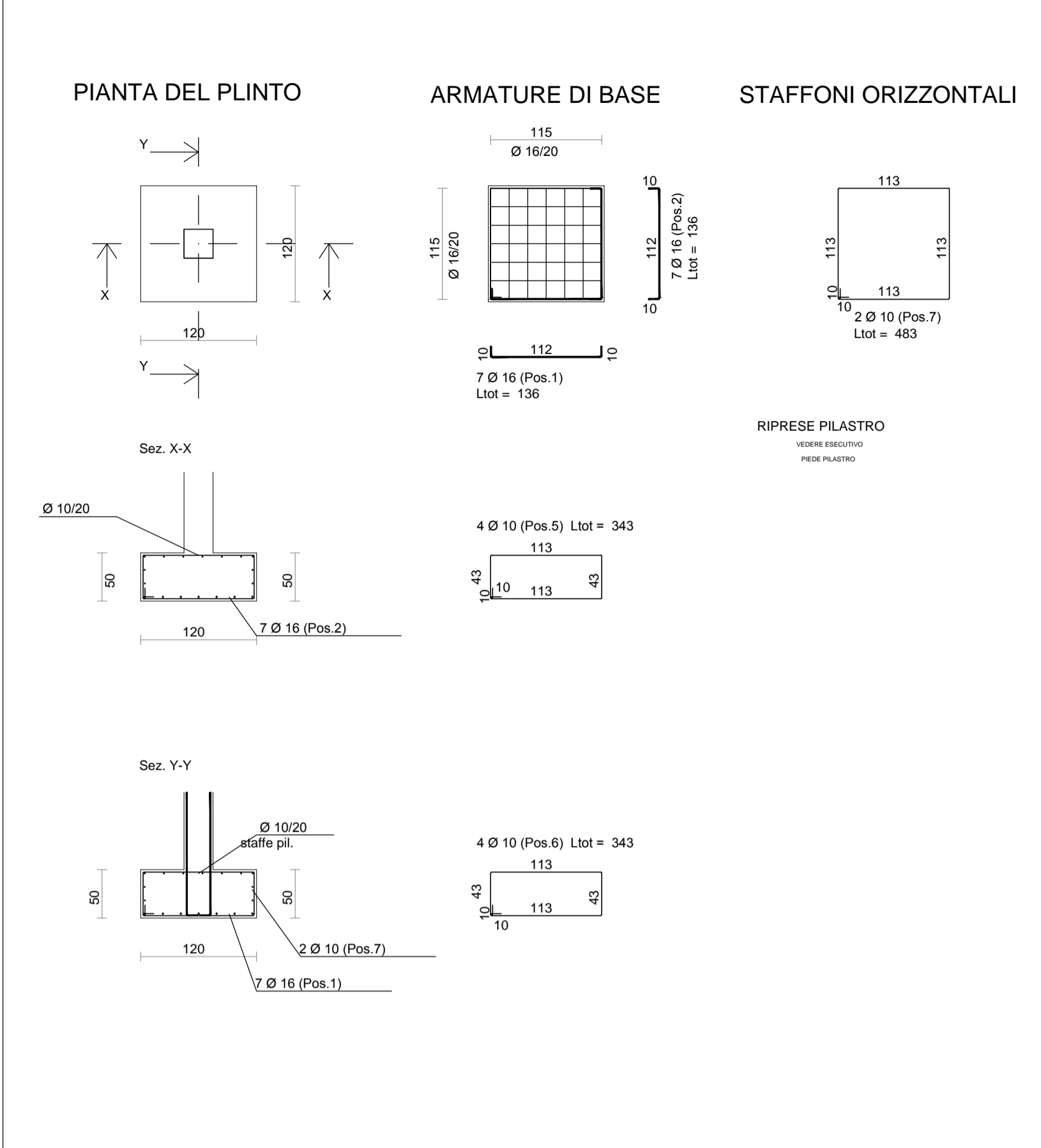
ZATTERA PLINTO N.ro 88-95-100 scala 1:50
