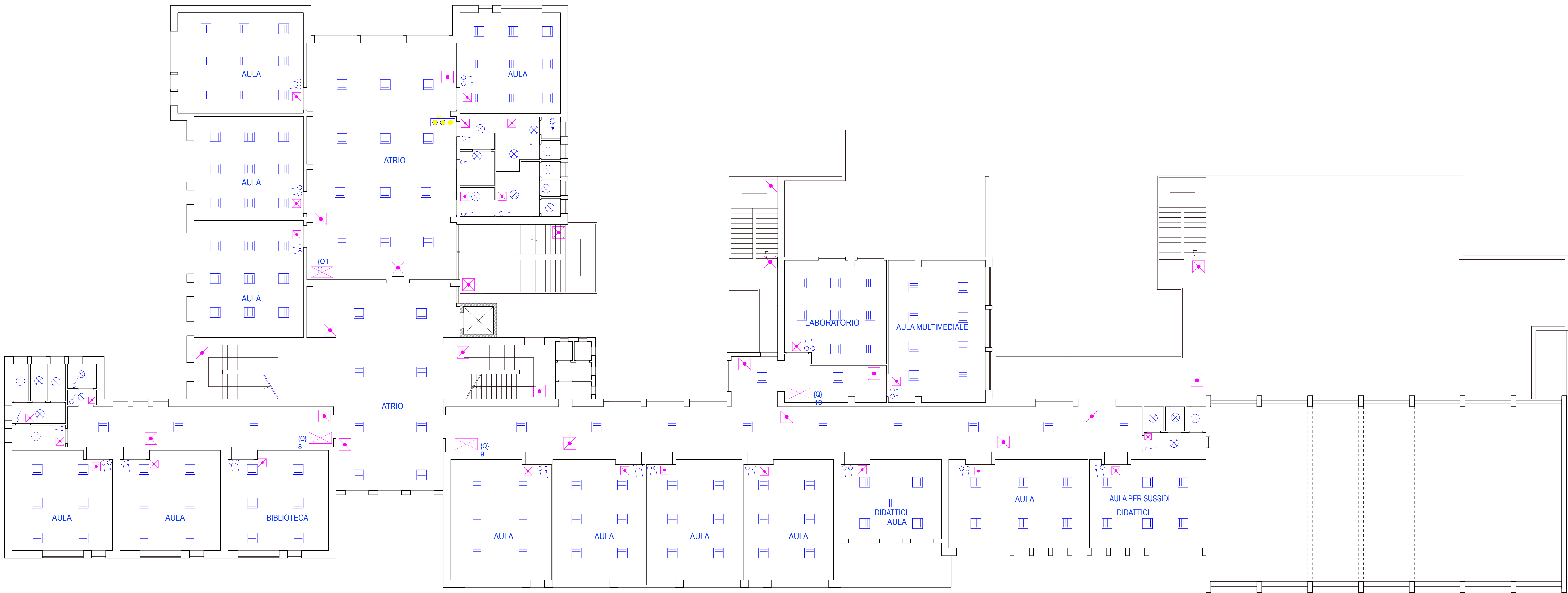
PIANTA PIANO PRIMO rappr. 1:100
